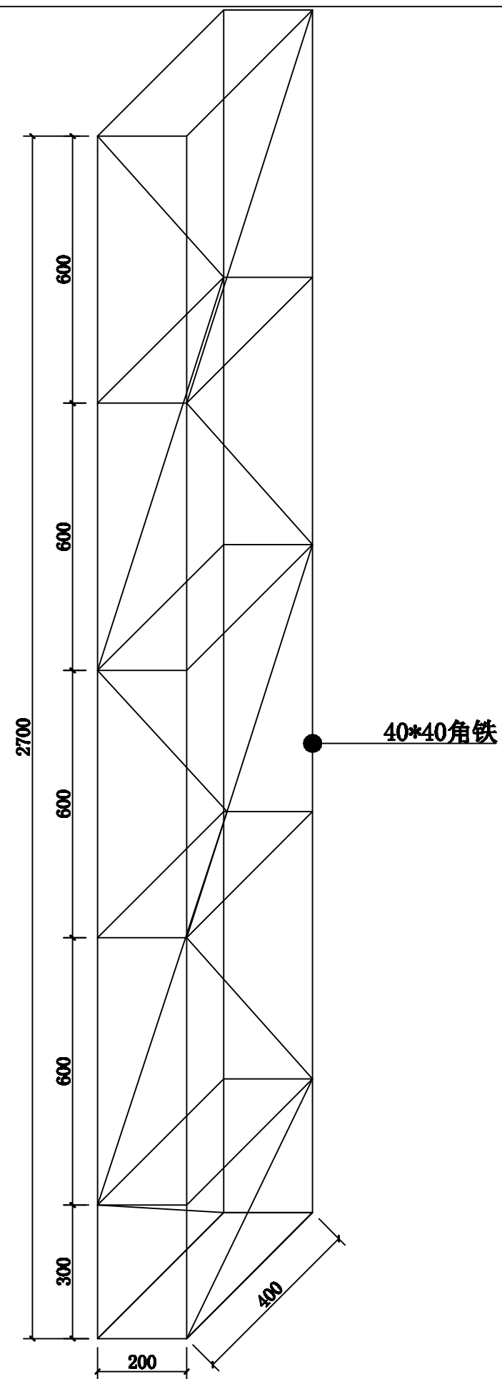
2.5米围蔽猪龙架大样图
